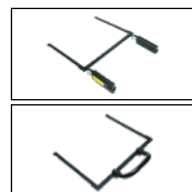
Seatfix-Adapter hinter dem Sitz (oben), Stabilisierungsbügel (unten)
